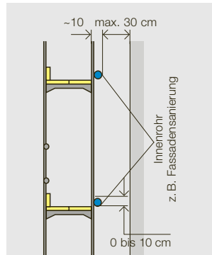
Bild 13: Innenrohre. Nur zulässig, wo keine Konsolgänge möglich sind
