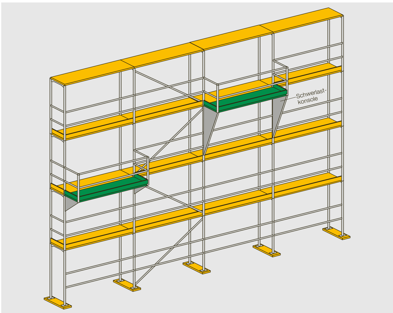
Bild 27: Versetzte Podeste für den Materialumschlag
