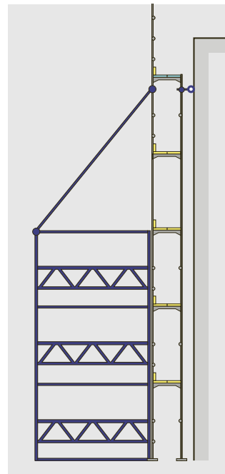
Bild 19: Beispiel Aussenabstützung mit querstehenden Gerüstfeldern
