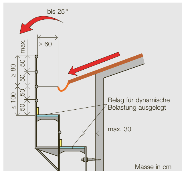
Bild 22: Seitenschutz eines Spenglergangs bei einer Dachneigung bis 25°
