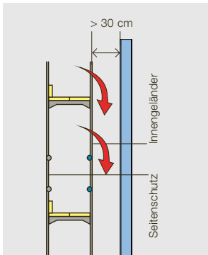
Bild 12: Innengeländer im Element- und Skelettbau
