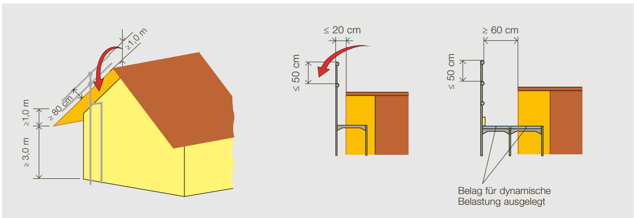
Bild 24: Giebelseitiger Seitenschutz
