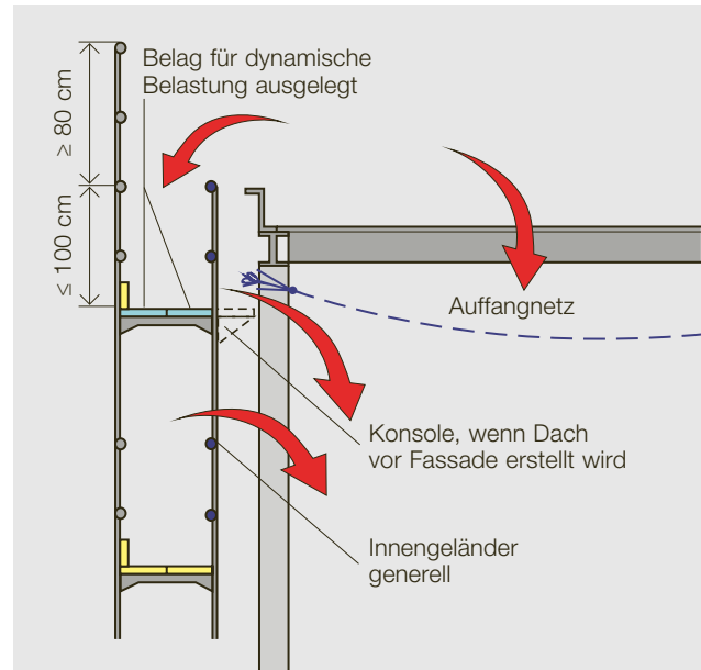
Bild 25: Montagebau
