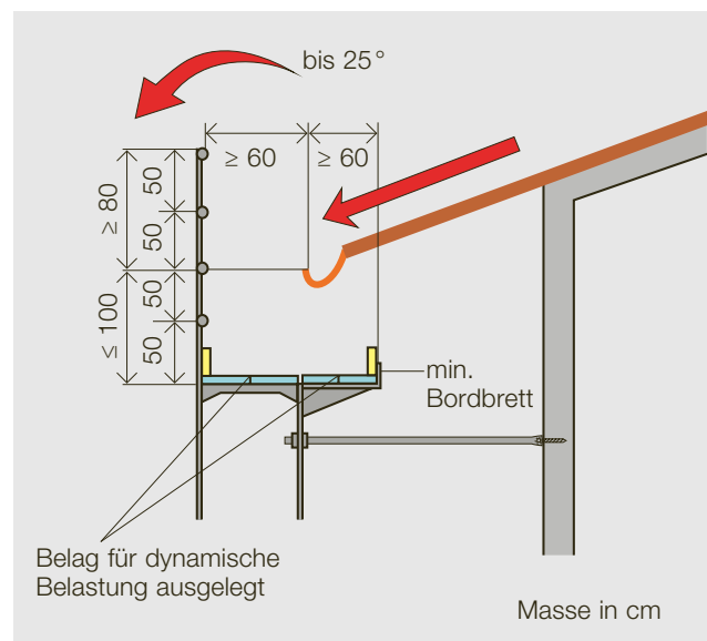
Bild 26: Traufrinne ersetzen, Ziegel auswechseln.
