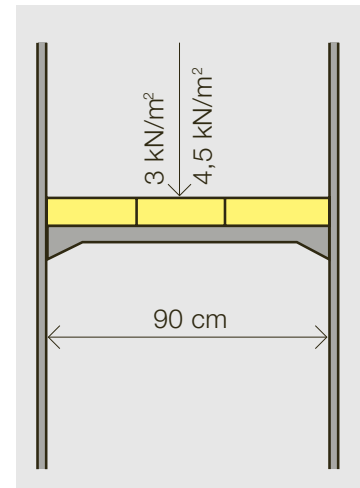
Bild 4: Maurergerüst bzw. Steinhauergerüst
