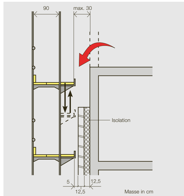
Bild 10: Nachträglich hochgezogenes Sichtmauerwerk
