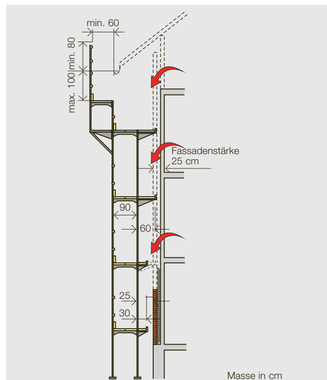
Bild 11: Nachträglich hochgezogenes Putzmauerwerk
