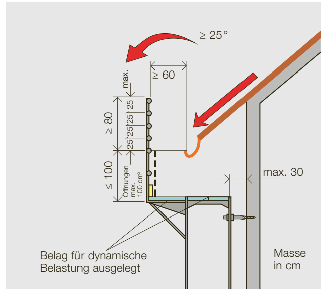
Bild 23: Spenglergang mit Dachdeckerschutzwand
