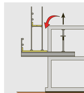
Bild 9: Auslegergerüst
