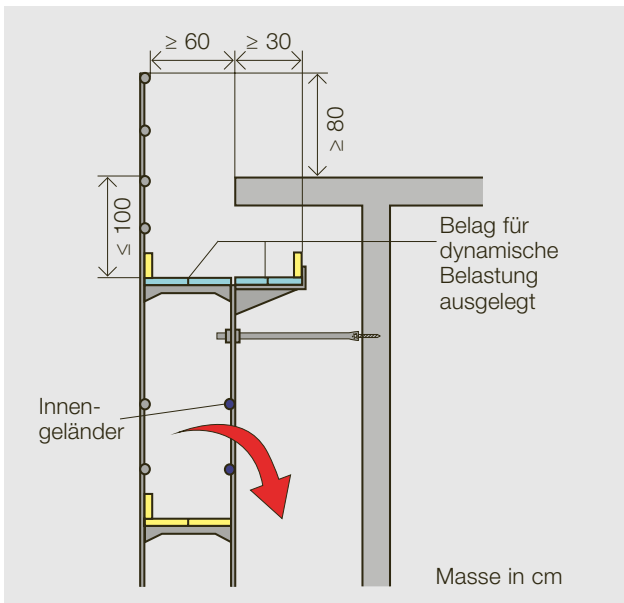
Bild 20: Spenglergang
