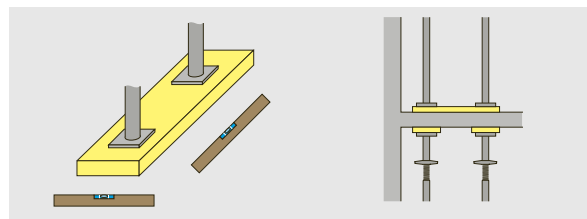
Bild 7: Konventionelle Fundamente
