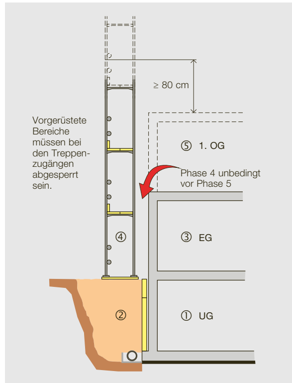
Bild 6: Vorgehensschritte 1 bis 5
