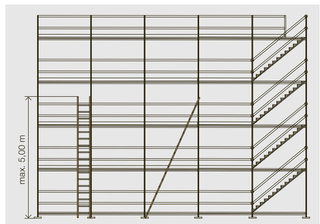
Bild 17: Leitern bis zu einer Höhe von höchstens 5 m
