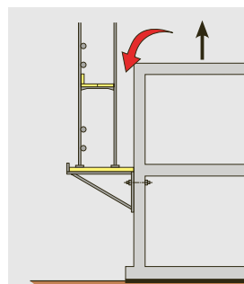
Bild 8: Konsolgerüst
