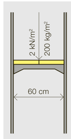
Bild 3: Verputz-/Malergerüst
