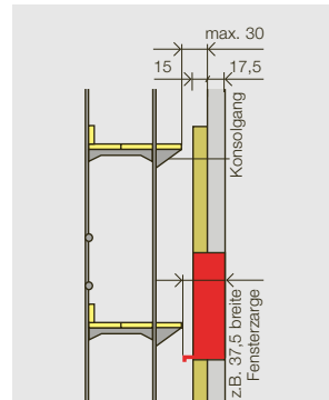
Bild 14: Konsolgänge
