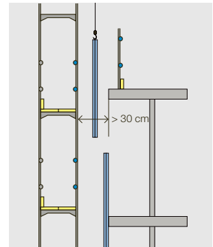
Bild 15: Versetzen von Fassadenelementen
