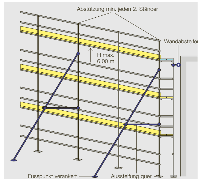
Bild 18: Aussenabstützung anstelle von Verankerungen
