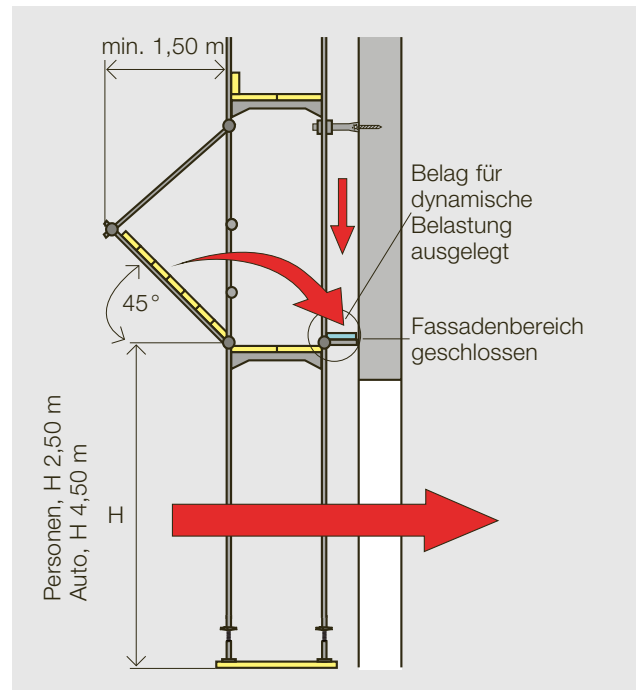
Bild 28: Schutz bei Durchgängen
