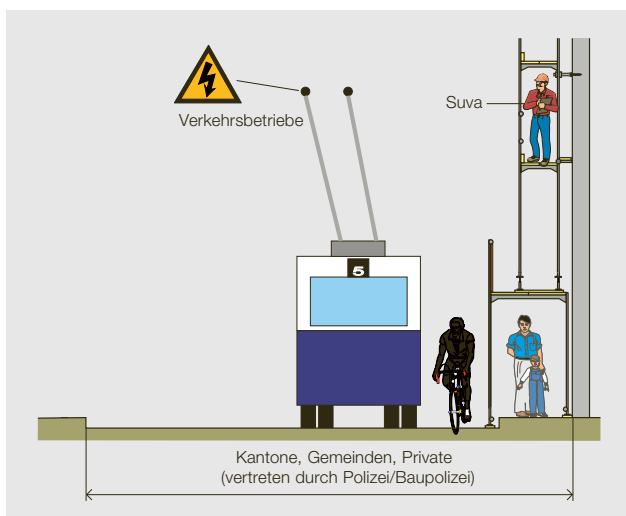
Bild 2: Schnittstelle Baustelle/öffentlicher Verkehr. Die Massnahmen sind mit den zuständigen Behörden abzusprechen.
